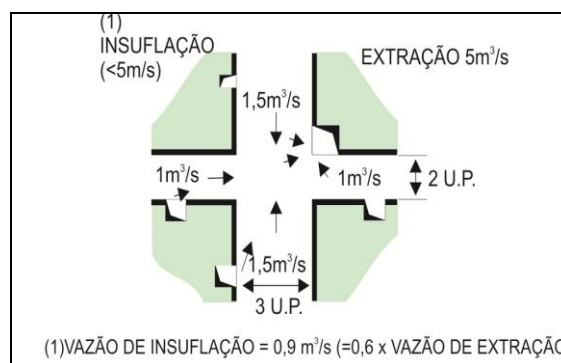
Figura 28 - Resumo geral de aberturas de extração de fumaça e entrada de ar em um pavimento
