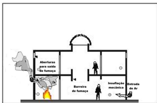
Figura 12 - Exemplo de controle de fumaça por extração mecânica e entrada de ar mecânica
