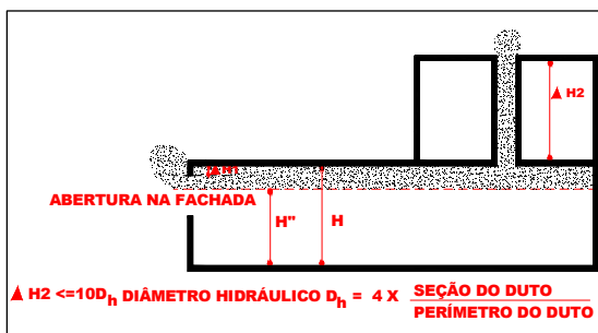
Figura 17 - Diâmetro hidráulico
